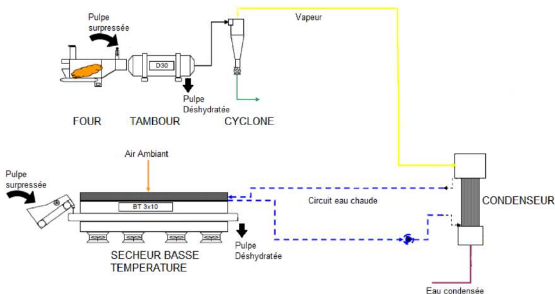
Figure 2 : Schéma de principe
