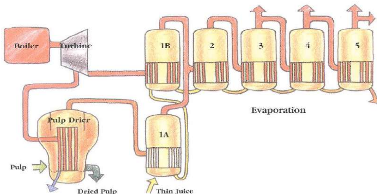
Figure 4 : Schéma d'intégration dans une sucrerie
